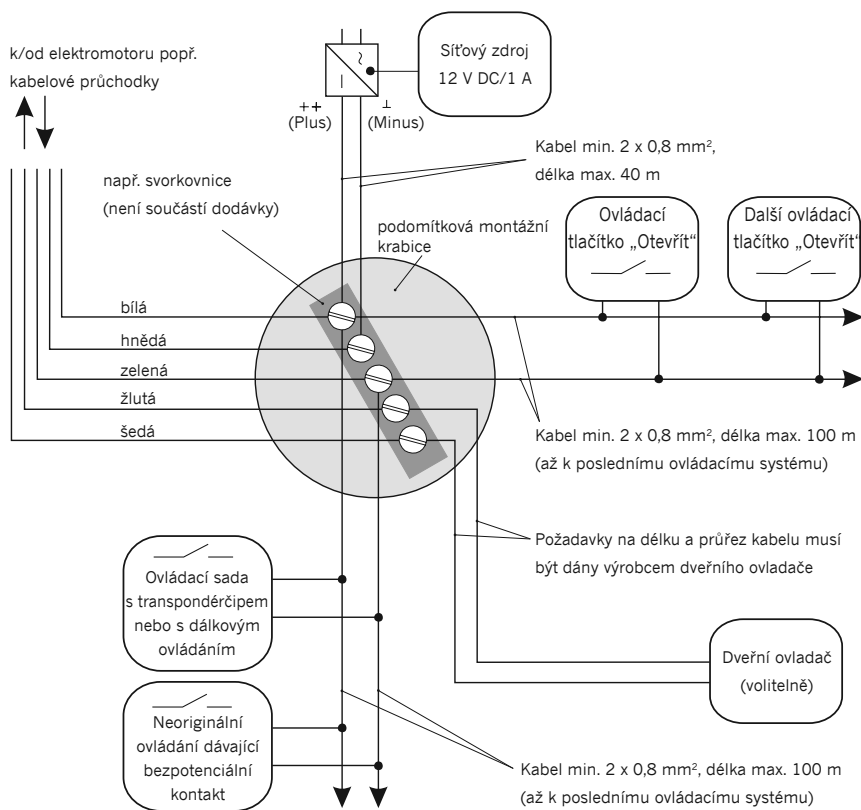
Obr. 3.3.1-1: Schéma zapojení
